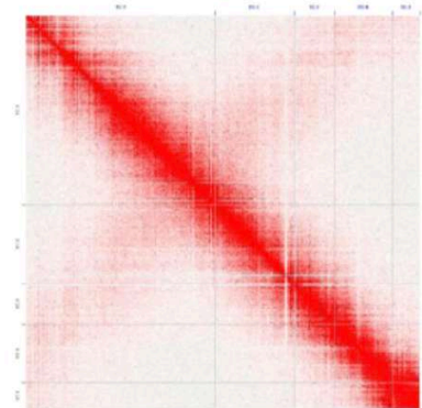
Chr 5C (612 Mb)
